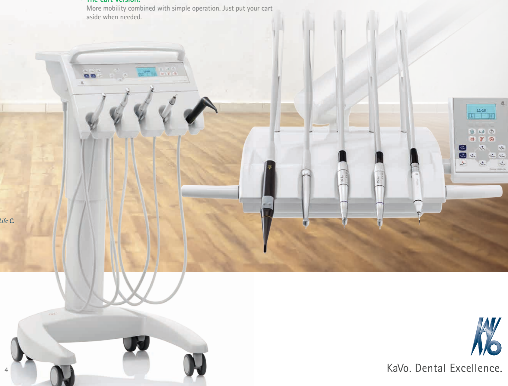
Swing-arm version KaVo Primus 1058 Life S.
